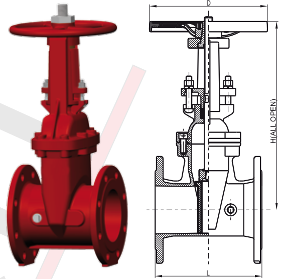
Fig . VIT-GTR-300
